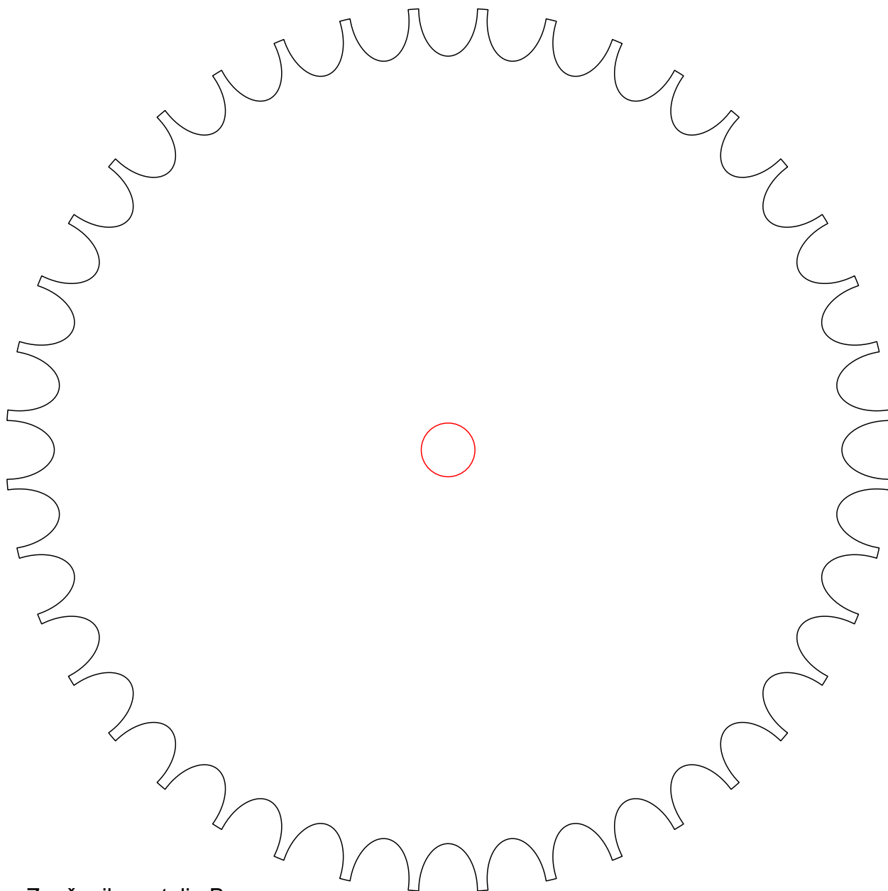
Zupčanik postolja B
